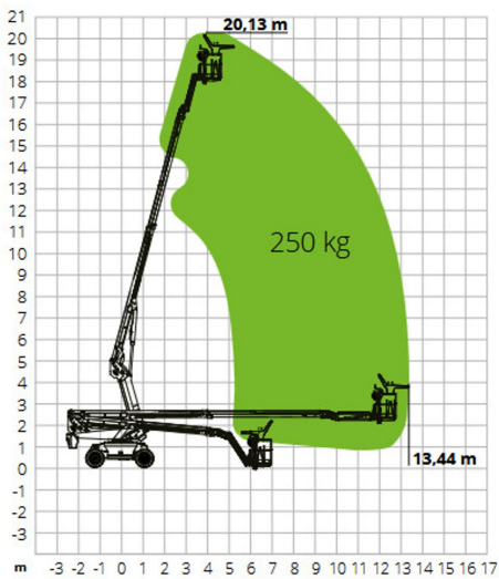
LASTDIAGRAMM
